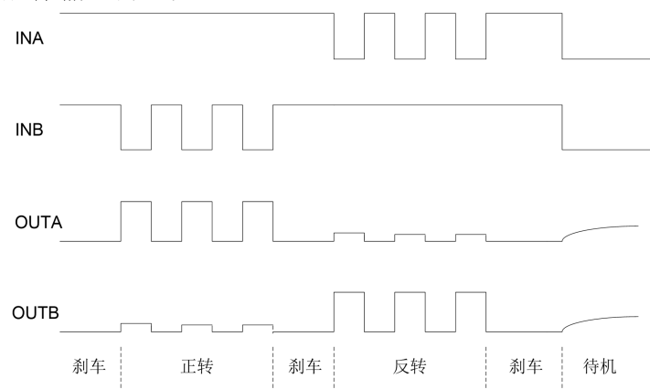
图4. 推荐输入方式时序图
