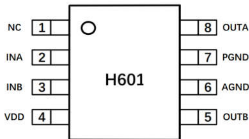
SOP8 H601
