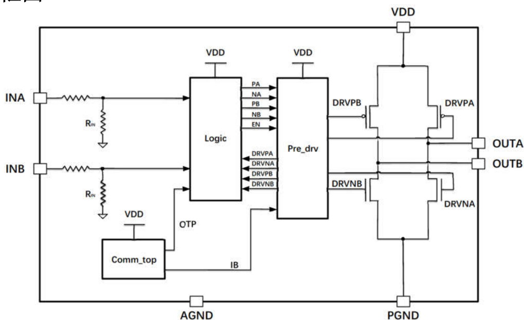
图 3. H601/H601A 系统框图
