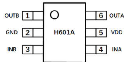
SOT23-6 H601A
