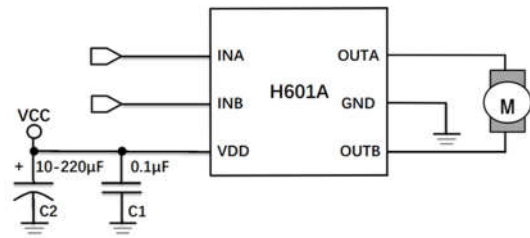
图 2. SOT23-6 典型应用电路图
