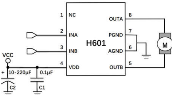
图 1. SOP8 典型应用电路图
